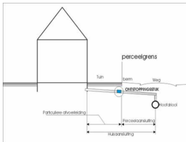
Figuur. Aansluiting op vrijvervalriolering
